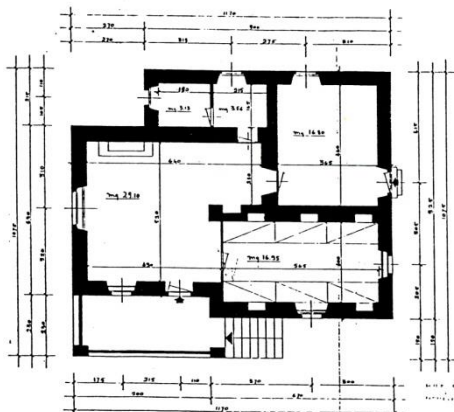
Fig. 1 PIANTE PIANO TERRA ESISTENTE
